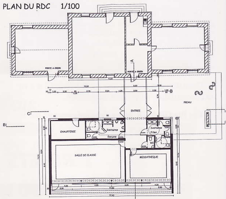
PLAN DU RDC 1/100
